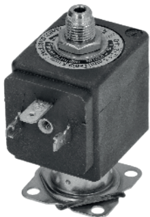
Ø 1,5 700175 V220/50/60 700175/11 V110 700175/24 V24/50/60
