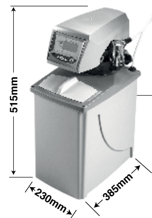
702534 VOLUMETRICO VOLUMETRIC GIX LT. 5
