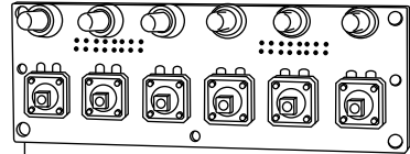
560064 PULSANTIERA VENEZIANO GR2/3 GICAR CODE 9.9.11.99G
