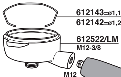
TAPPO CROMATO CHROMATE PLUG
